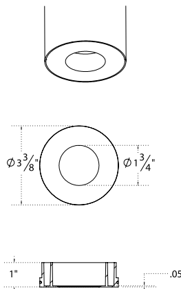
B3R-315-DC-TL
